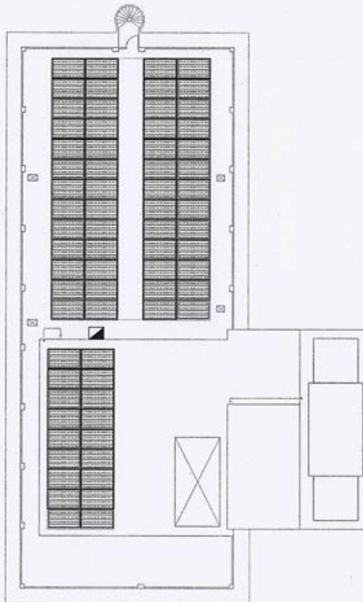
แปลนชั้นดาดฟ้าอาคารจำลองฯ สำหรับติดตั้งระบบผลิตไฟฟ้าจากพลังงานแสงอาทิตย์
