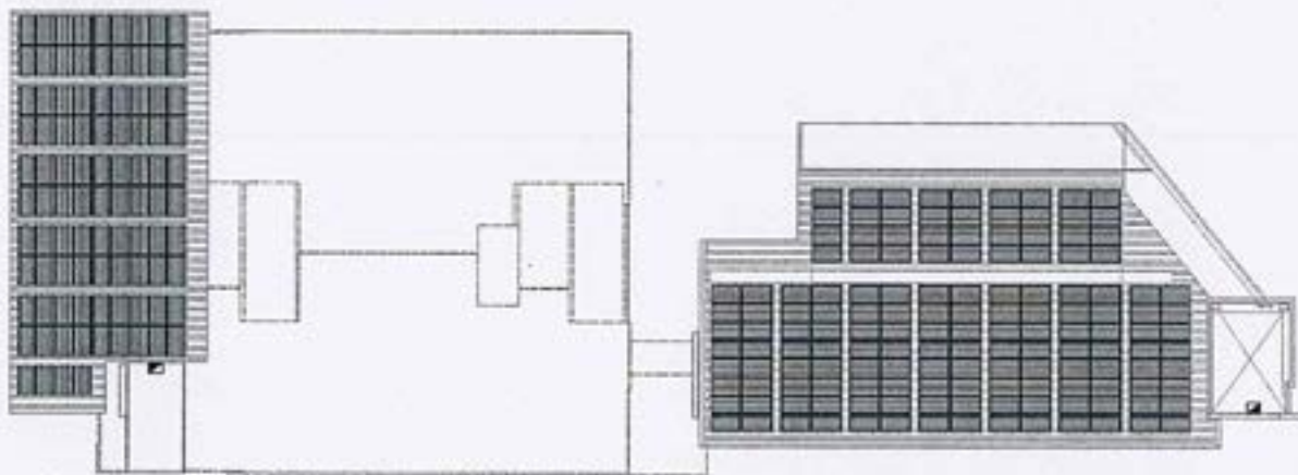
แปลนหลังคาอาคารเฉลิมมา 60 ปี สำหรับติดตั้งระบบผลิตไฟฟ้าจากพลังงานแสงอาทิตย์
